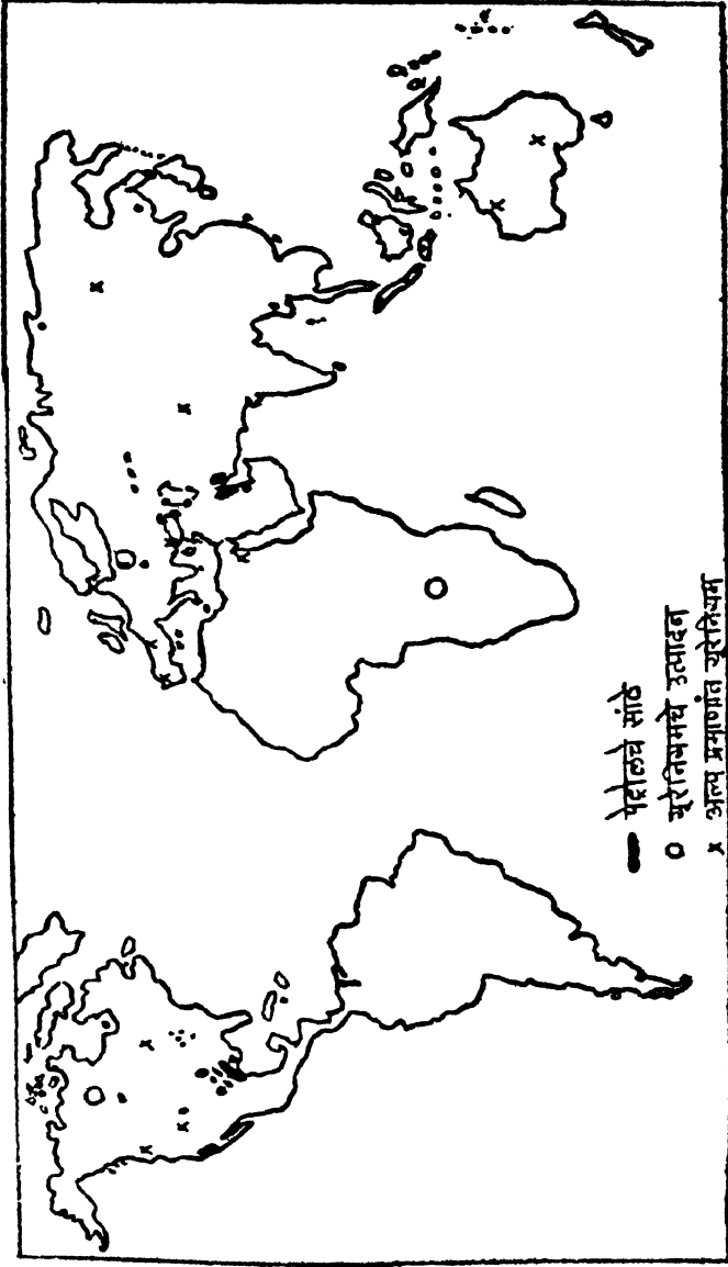
नकाशा २ जगातील पेट्रोल व युरेनियमचे सांठे.
